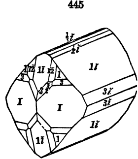
Danaite.
